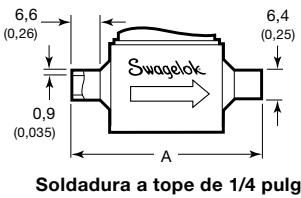
Soldadura a tope de 1/4 pulg
